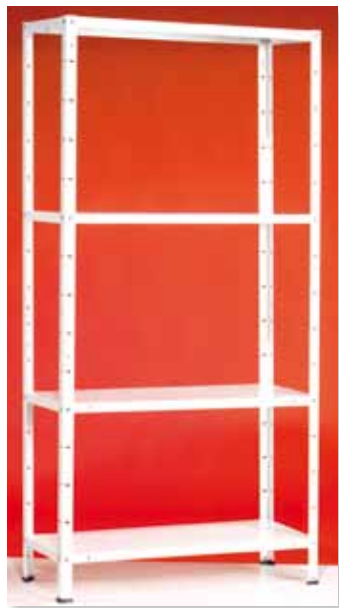
Módulo estantería 4 bateas 75 x 30 x 150 cms. Cod: 21030500 ORYXI
